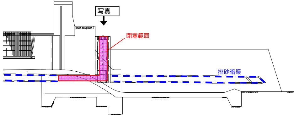
側面図
